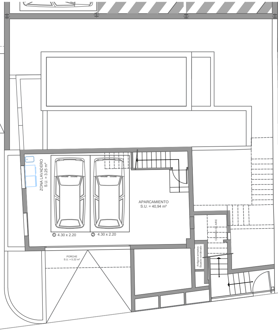
PL. SEMISOTANO
