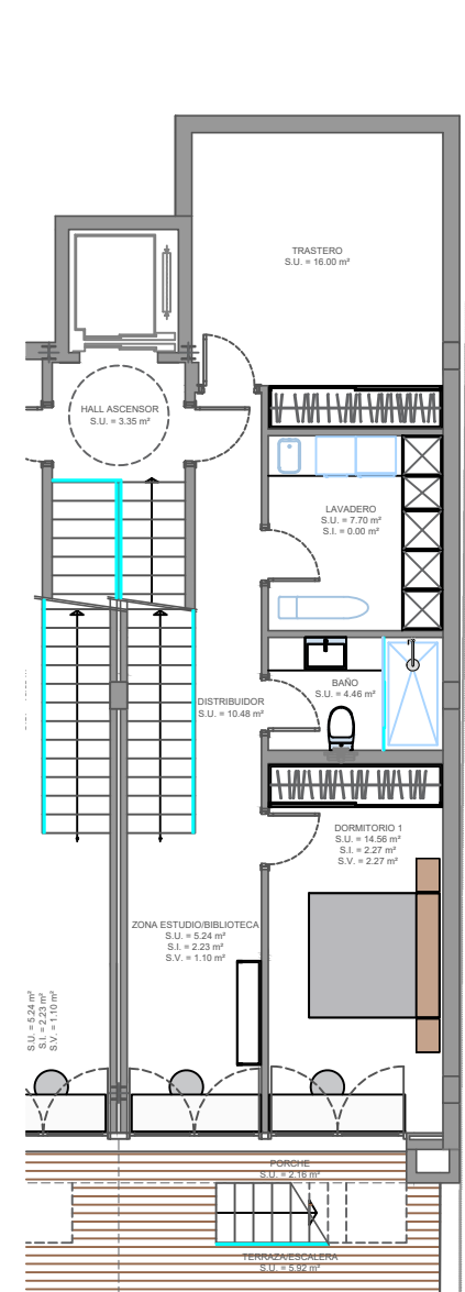
PL. SEMISOTANO
